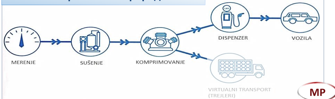
Шема компримовања природног гаса
